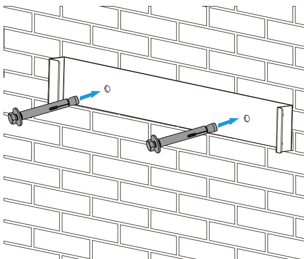
Рис. 4.5 Установка монтажной скобы
