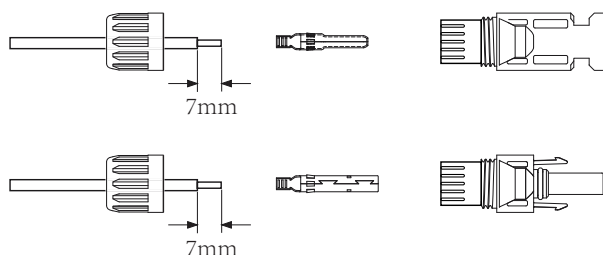
Рис. 5.3 Разбор коннектора
