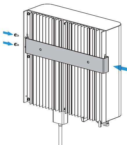
Рис. 4.6 Монтаж инвертора
